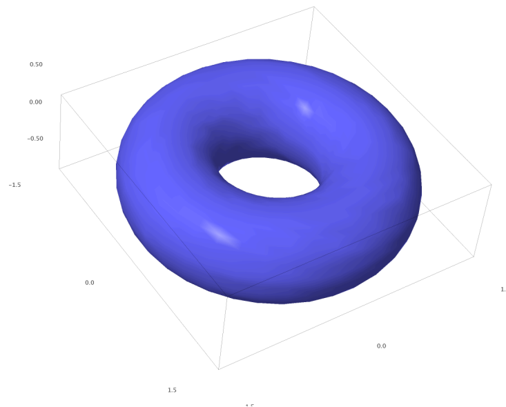
FIGURE 8 – Un tore complexe de dimension 1
